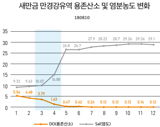
가로축(수심m), 세로축(농도) : 수심 3~4m 지점에서 용존산소와 염도의 급격한 변화가 있는 수심대가 새만금 전 수역에 동일하게 형성되어 있다.
